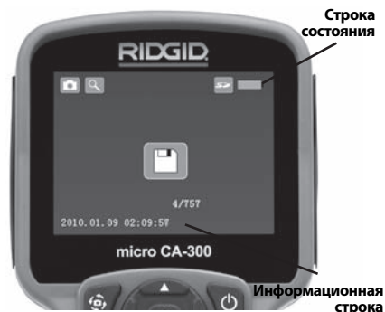
Рис. 13 - Рабочий экран
